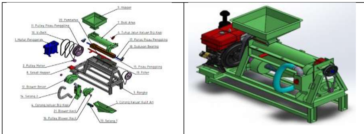
Gambar 4. Mesin Wet Hulling Kopi
