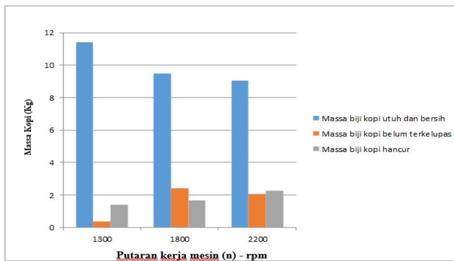
Gambar 7. Grafik hasil pengujian mesin wet hulling
